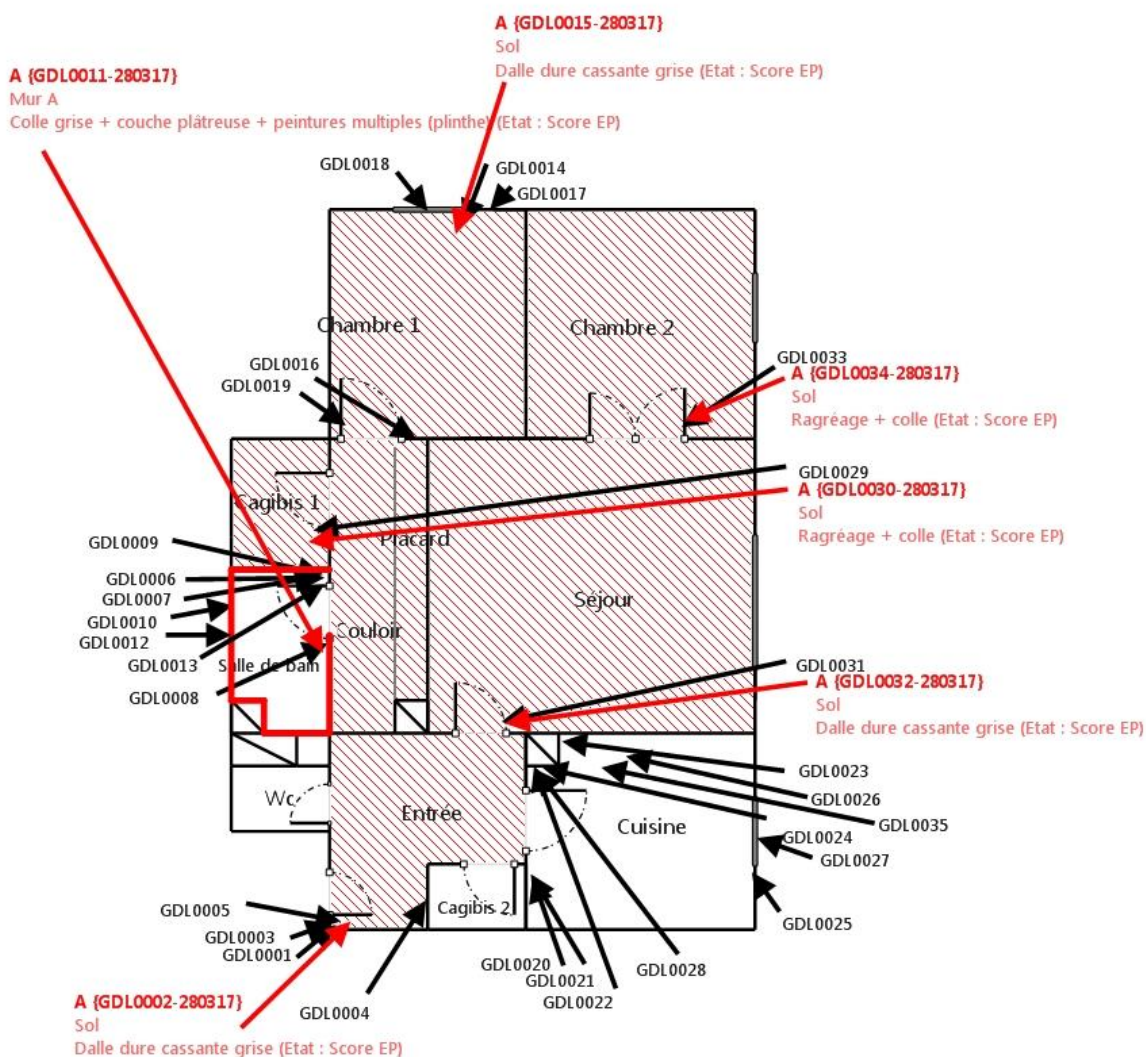
Planche (croquis) de repérage technique effectué par le cabinet : ALLODIAGNOSTIC, auteur : Geraud DE LAFFON Dossier n° 862738 du Adresse du bien : 4 SQUARE PAUL ALGIS ESC AD 50LAD0404 (50LAD0404) 77360 VAIRES SUR MARNE
